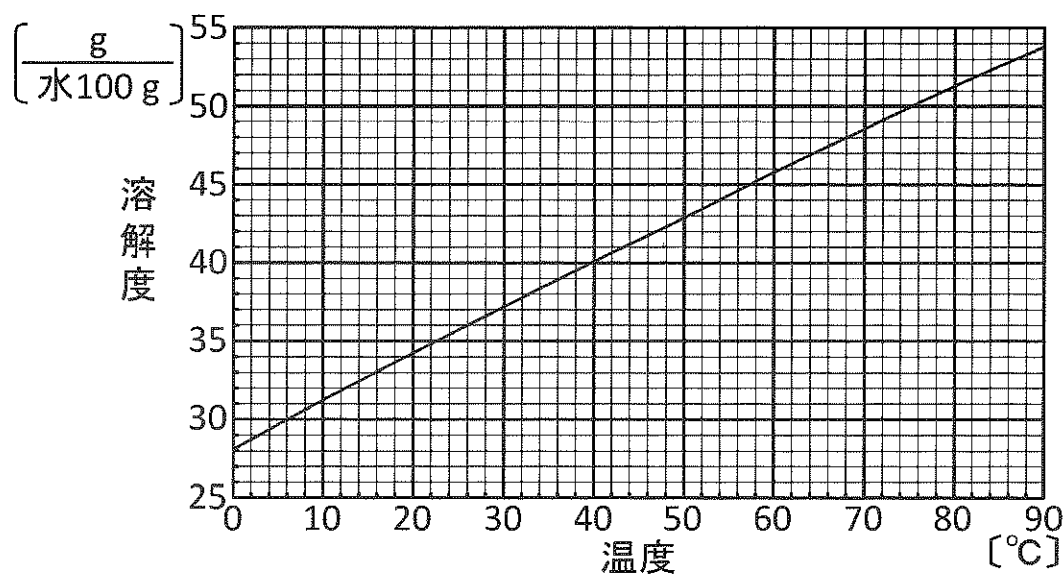
図1 塩化カリウムの水への溶解度曲線
