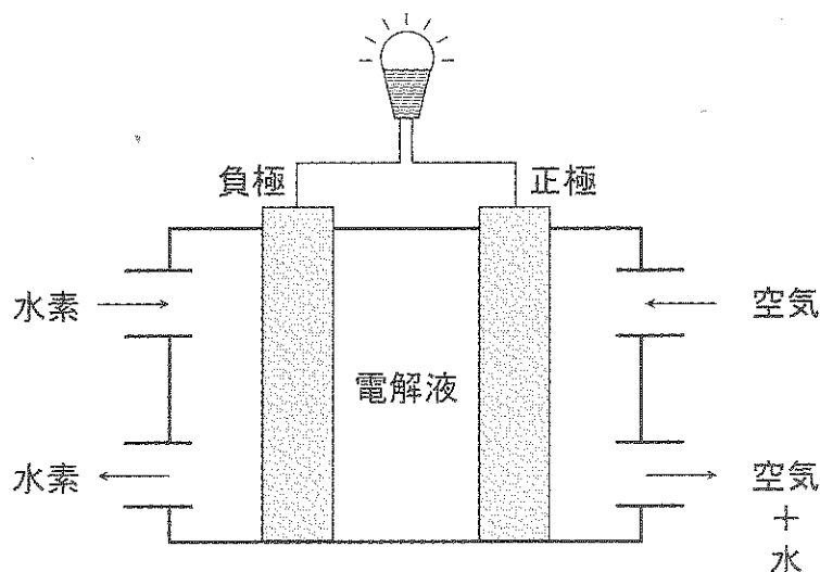
図1 燃料電池
