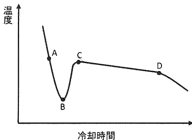
図2 冷却曲線
